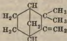
Camphene.
